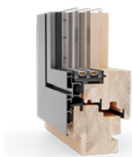
Gemini Quadrat FB Standaardprofiel (met uitsparing)
