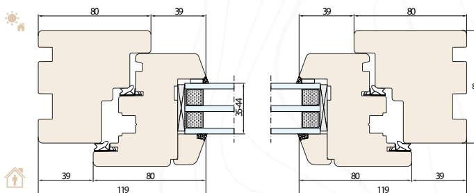
NATURO 80 SYSTEEM HORIZONTAAL DOORSNEDE B-B
