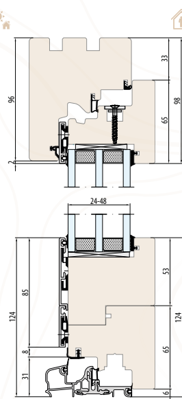
ESPERIA LIFE 80 SYSTEEM enkele balkondeur met lage drempel
