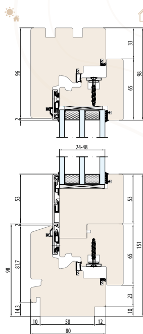
ESPERIA LIFE 80 SYSTEEM enkele balkondeur met hoge drempel
