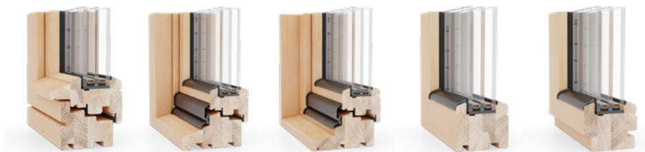
Belgisch profiel B (zonder uitsparing)
