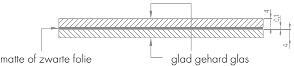
Standaard VSG/ESG gelijmd en gehard glas, melkachtig of zwart
