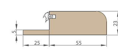
Hardhouten drempel
