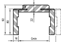
OR/ORC sectie met hoek. T80
