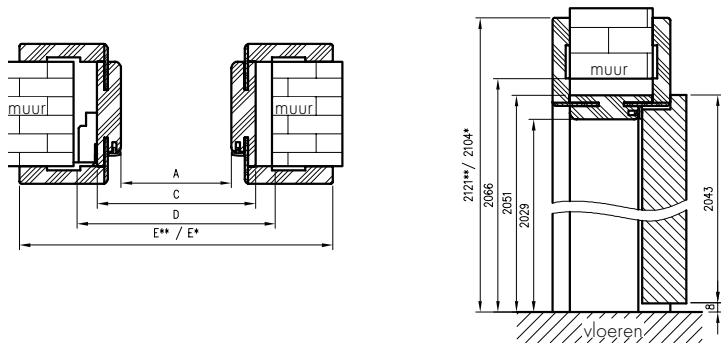
Hoogteafmetingen voor sponningvrije deuren
