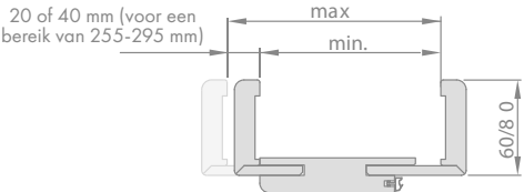
INSTELBEREIK VAN HET VERSTELBARE FRAME
