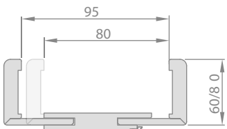
VERSTELBAAR FRAME BEREIK 80-95MM
