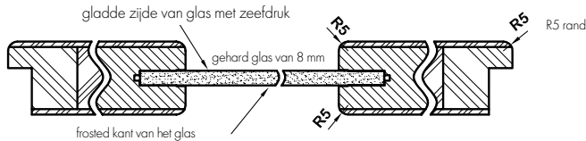
DEUR HORIZONTALE SECTIES VETRO D1
