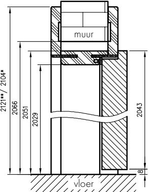
Verticale doorsnede van sponningdeur met OR
