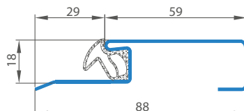
Roestvrij stalen drempel
