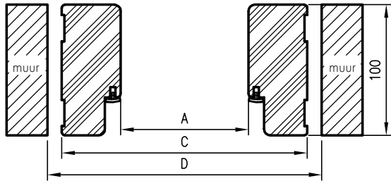
Hoogteafmetingen voor sponningvrije deuren
