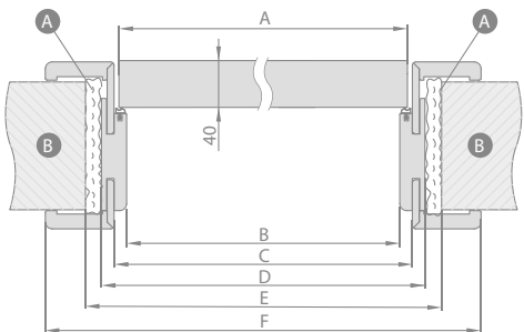
SCHEMA VERSTELBAAR FRAME
